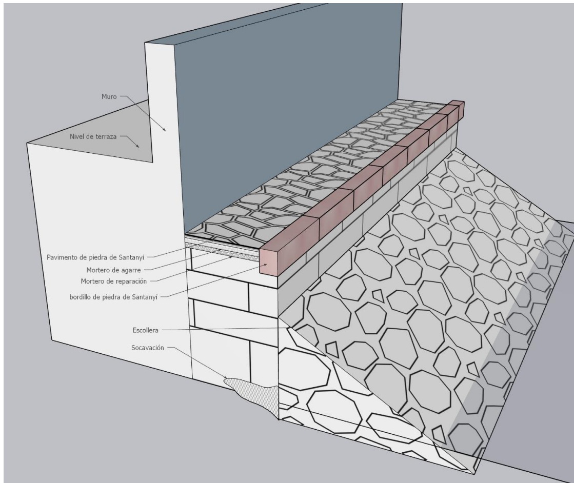
Il·lustració 15: esquema de una actuación en una sección con varios tipos de daños. Puede haber secciones en las que no sea necesario el vertido de escollera.
