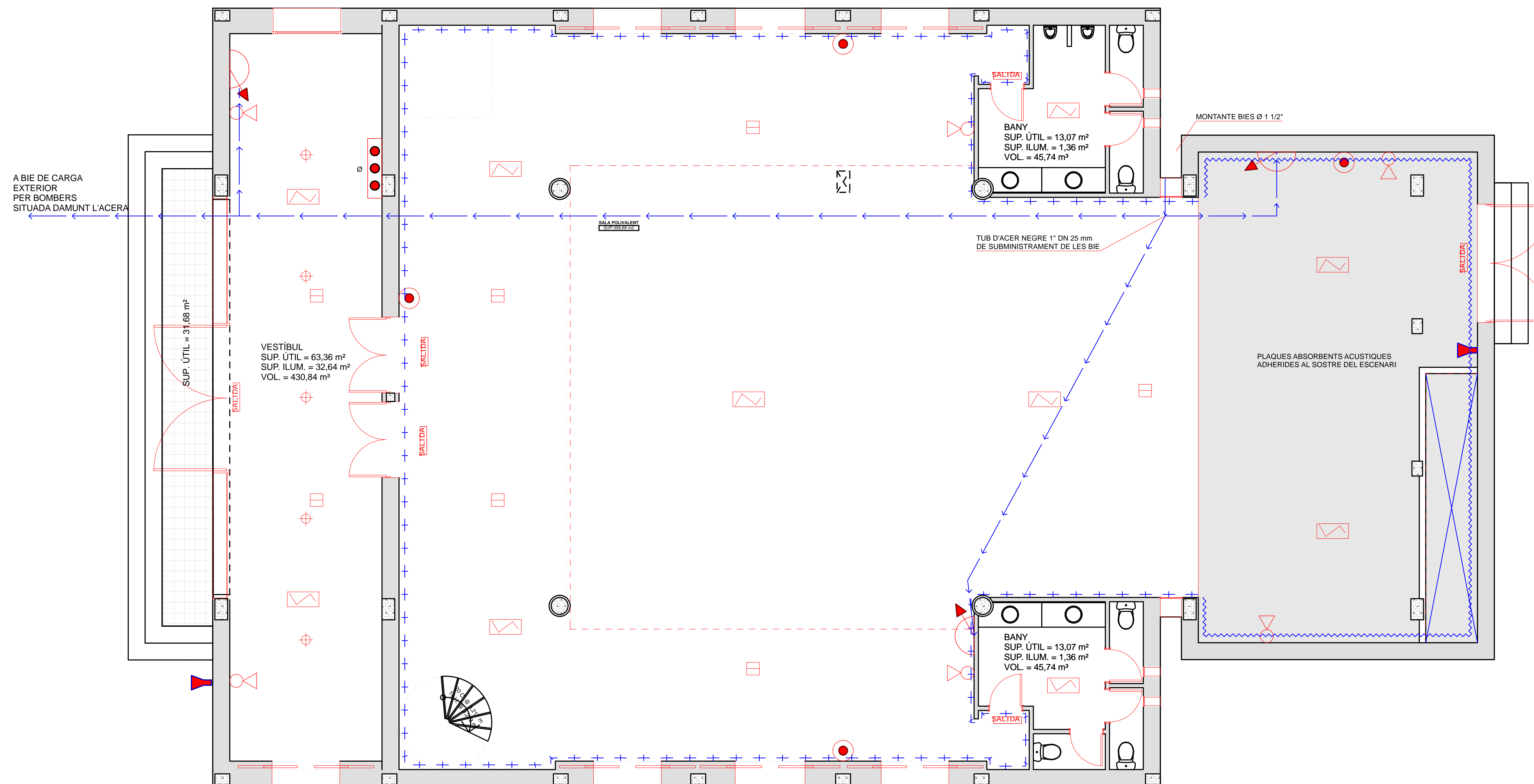
PLANTA BAJA SUP. CONSTRUÏDA 500,44 m²
